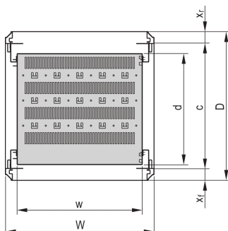
Ripiano Varistar 19", fisso, 75 kg.
